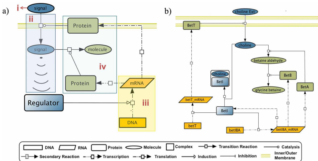
(a) El concepto genérico de Unidad GENSOR incluye 4 componentes: (i) la señal, (ii) la transducción de la señal mostrada en azul, (iii) el switch genético en amarillo y (iv) la respuesta mostrada en verde. (b) Unidad GENSOR de Beti. Ejemplo de un GENSOR basado en un regulador transcripcional microbiano.
